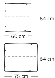
Faltkissen (Rücken) Foldable back cushion
