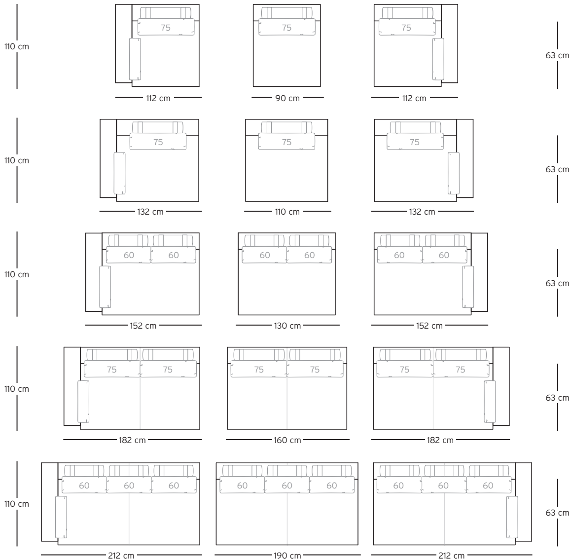
Elemente mit Armlehne links Elements with armrest left
